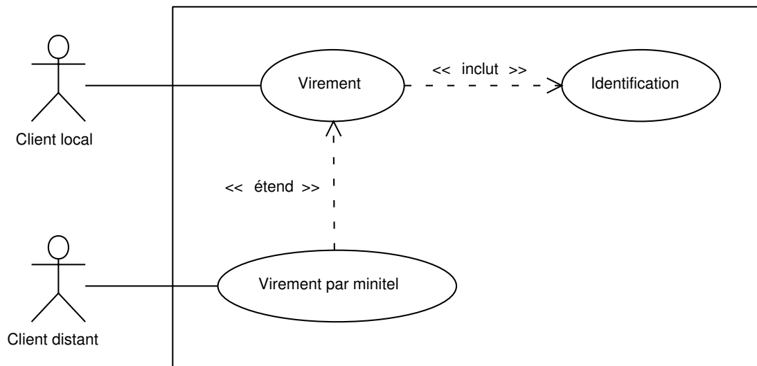
FIG. II. 7 – Diagramme de cas d'utilisation pour un système de virements bancaires
