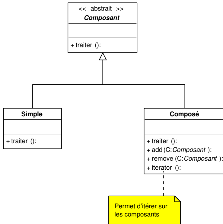
FIG. V. 2 – Diagramme de classes du patron Composite
