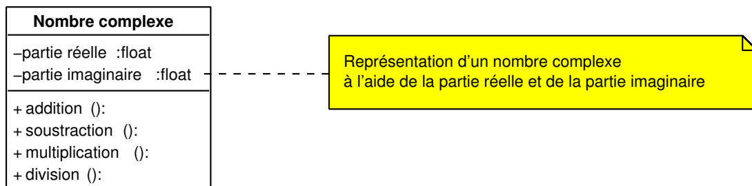
FIG. II. 14 – Classe des nombres complexes ; implantation avec parties réelle et imaginaire
