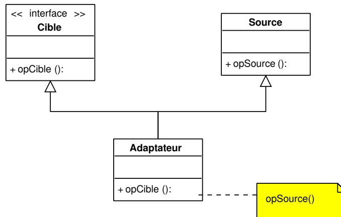
FIG. V. 4 – Patron Adaptateur, par héritage
