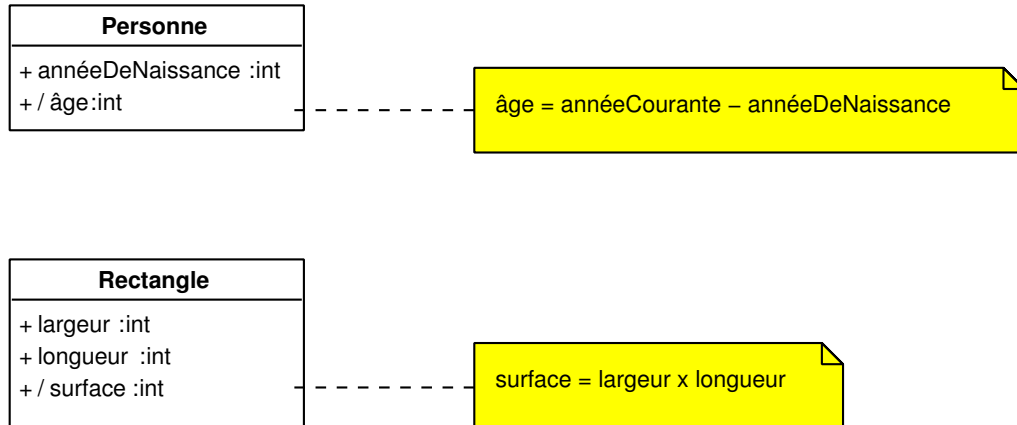
FIG. II. 10 – Exemples d’attributs dérivés
