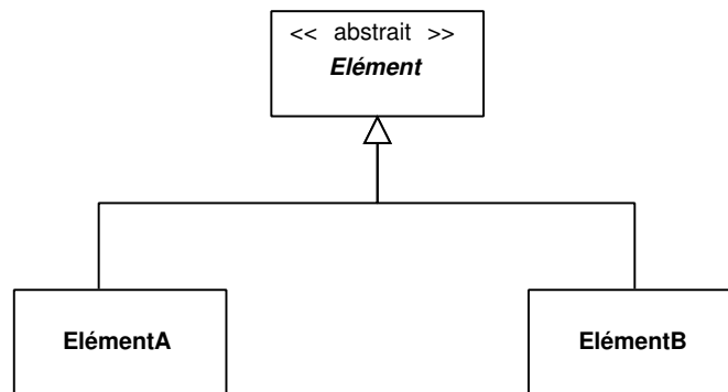
FIG. V. 15 – Hiérarchie Elément pour le patron Visiteur
