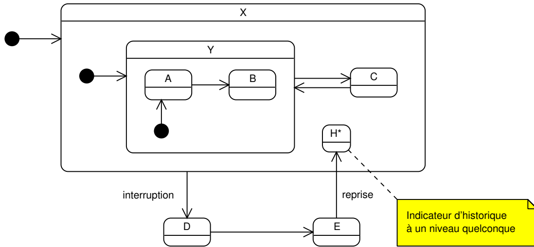
FIG. II. 75 – Indicateur d'historique à niveau quelconque
