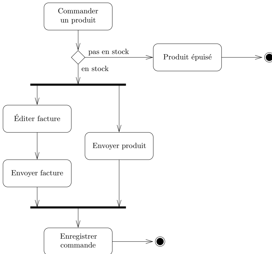
FIG. II. 78 – Diagramme d'activités pour une commande de produits
