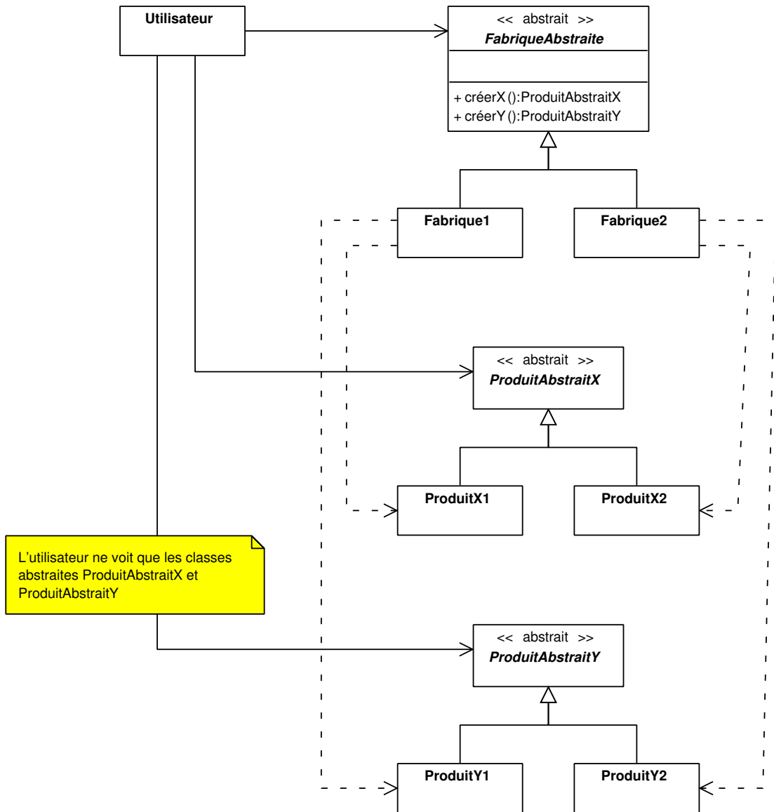
FIG. V. 1 – Diagramme de classes du patron Fabrique Abstraite
