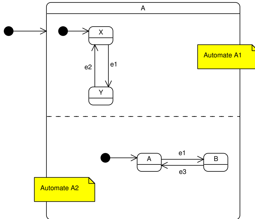
FIG. II. 76 – L'état A contient deux automates qui s'exécutent en parallèle
