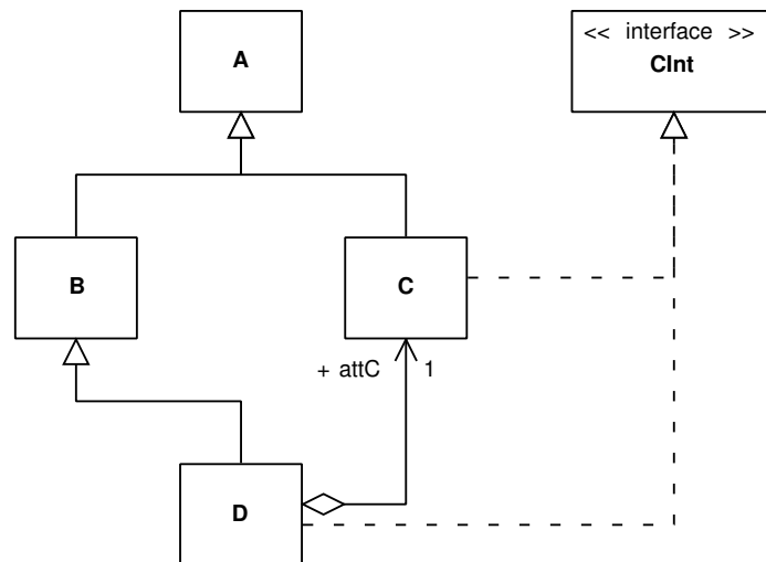
FIG. VI. 16 – Héritage multiple, simulé par délégation et interface
