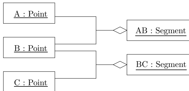
FIG. II. 34 – Diagramme d'objets modélisant les segments AB et BC
