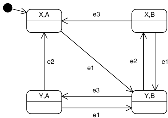
FIG. II. 77 – Automate « aplati » équivalent
