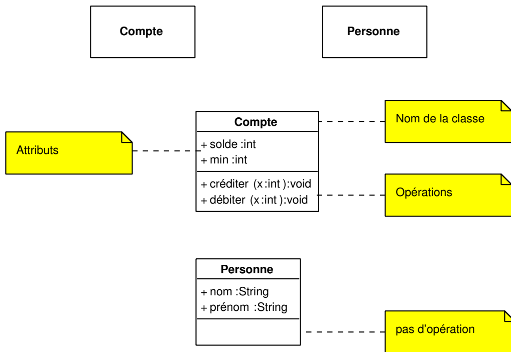
FIG. II. 9 – Représentation des classes Compte et Personne
