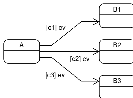
FIG. II. 70 – Transitions gardées, étiquetées par le même événement
