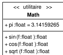
FIG. VI. 1 – Classe utilitaire Math
