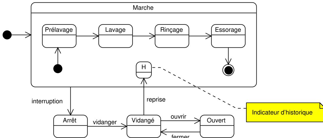
FIG. II. 74 – Diagramme d'états-transitions d'une machine à laver
