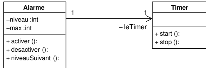
FIG. VI. 17 – Diagramme de classes de l'alarme
