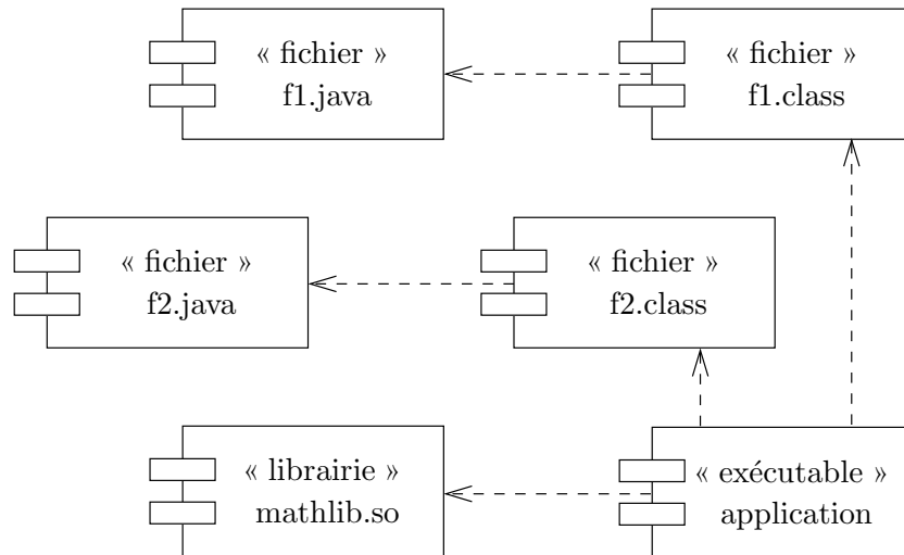
FIG. II. 79 – Diagramme de composants d'une application
