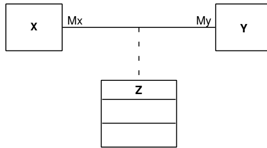
FIG. II. 26 – Multiplicités d'une classe-association
