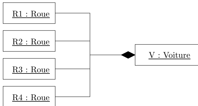
FIG. II. 38 – Un diagramme d'objets correspondant au diagramme de classes figure II. 37
