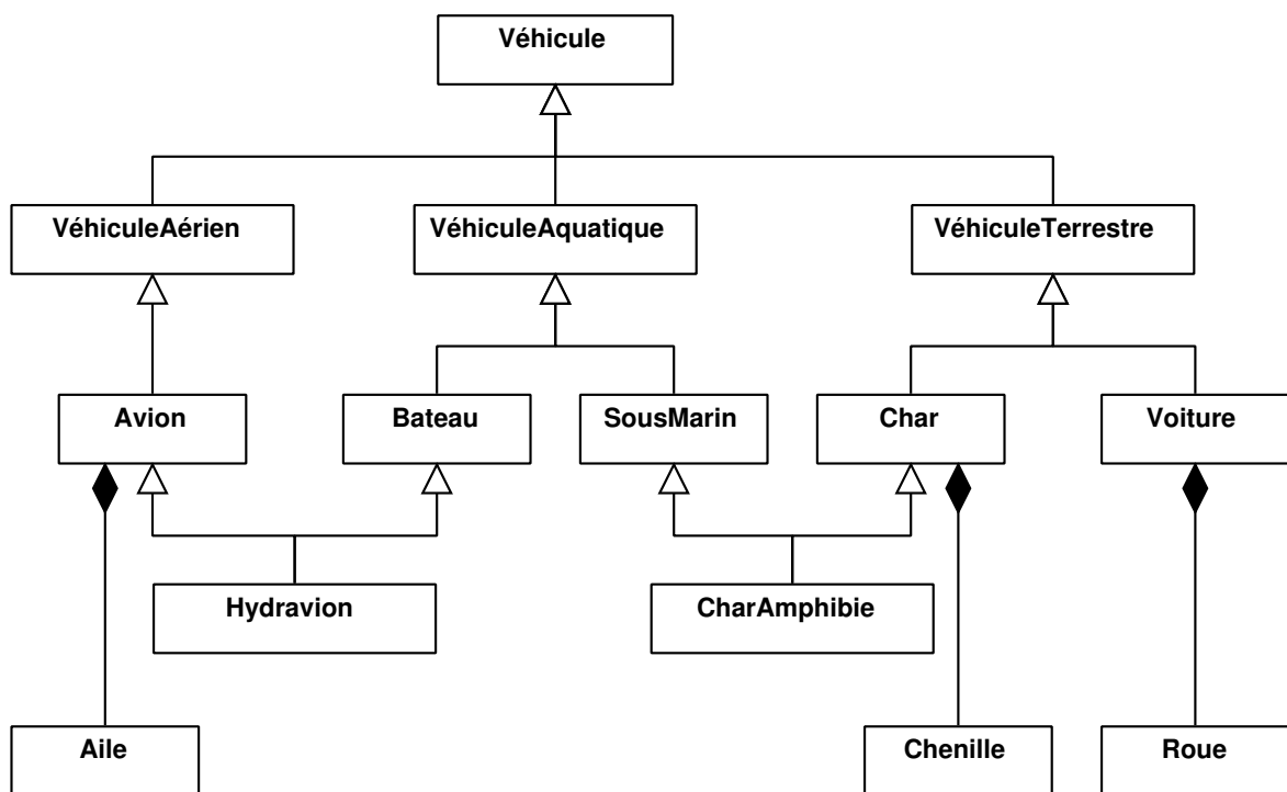
FIG. II. 44 – Hiéarchie de classes pour différents types de véhicules
