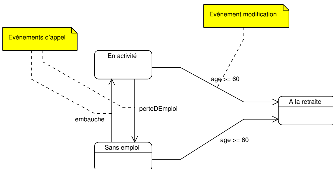
FIG. II. 66 – Diagramme d'états-transitions associé à la classe Personne
