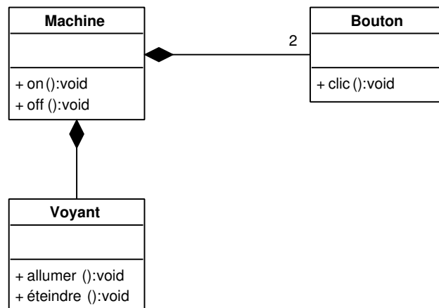
FIG. II. 67 – Diagramme de classes de la machine
