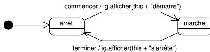
FIG. VI. 23 – Diagramme d'états-transitions de la classe Activité
