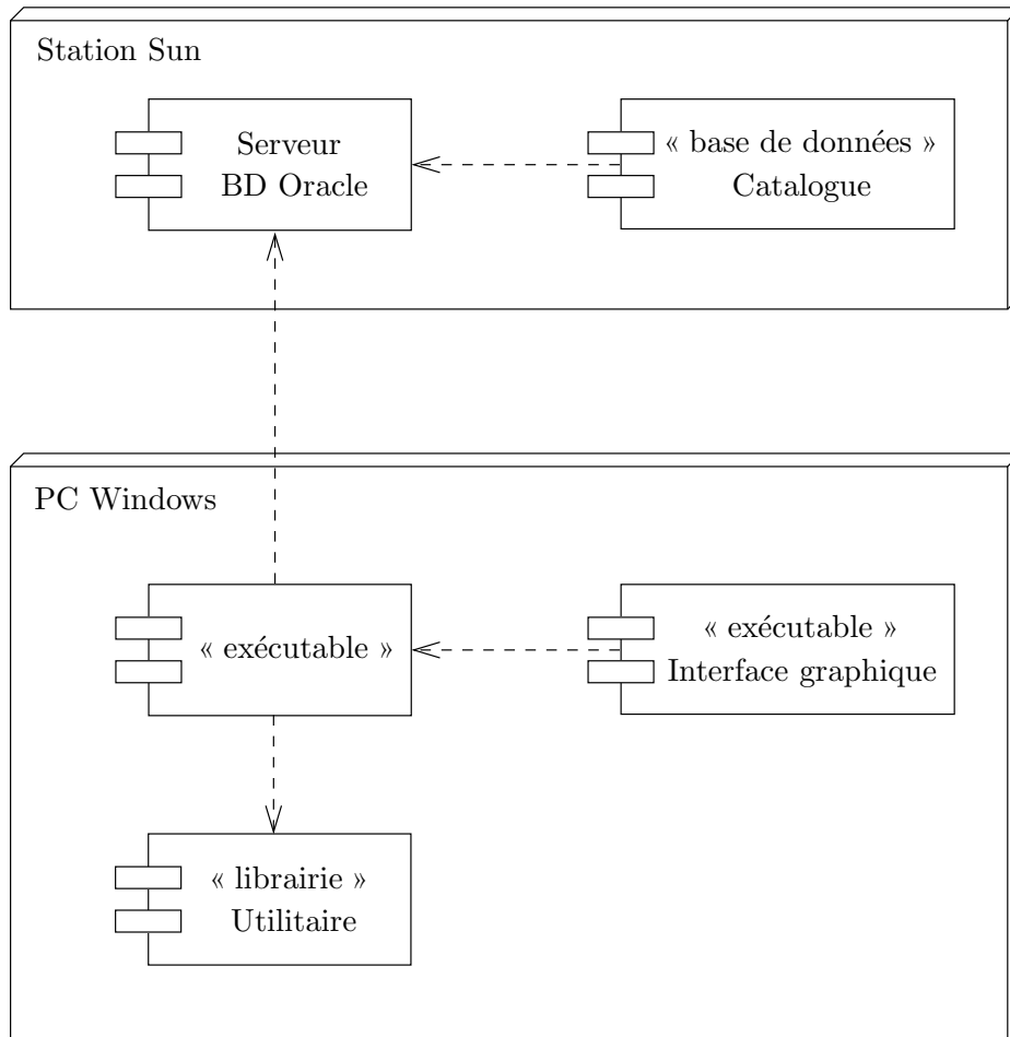
FIG. II. 81 – Diagramme de déploiement d'une application
