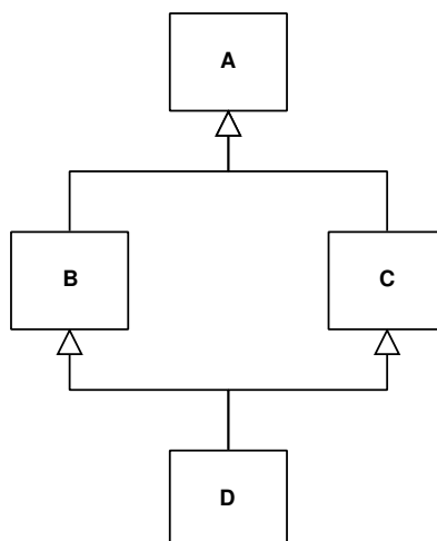
FIG. VI. 14 – Classe A héritée dans D par deux chemins
