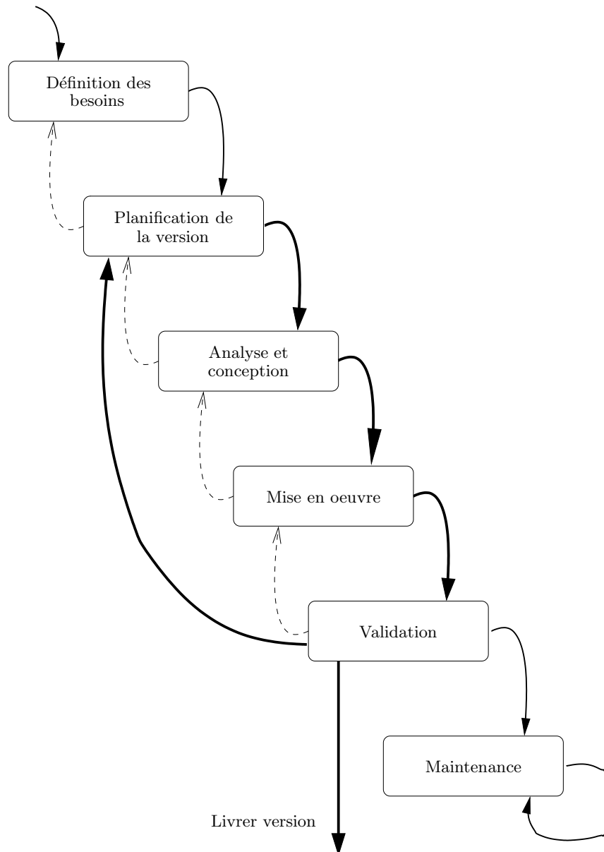
FIG. I. 4 – Modèle du cycle de vie incrémental
