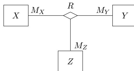
FIG. II. 40 – Association ternaire entre les classes X, Y et Z
