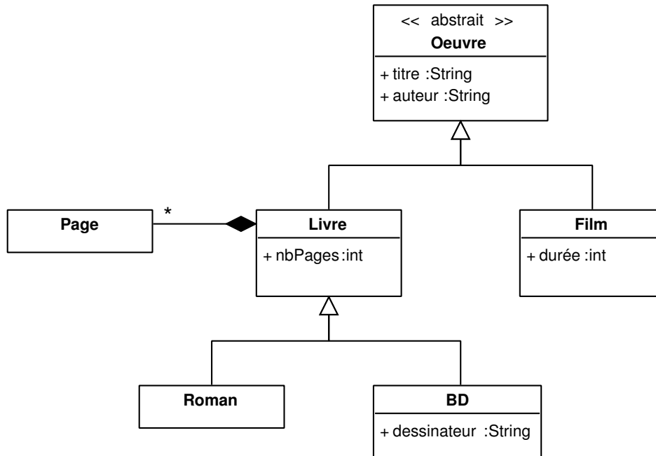
FIG. II. 47 – Hiérarchie de classes pour des œuvres
