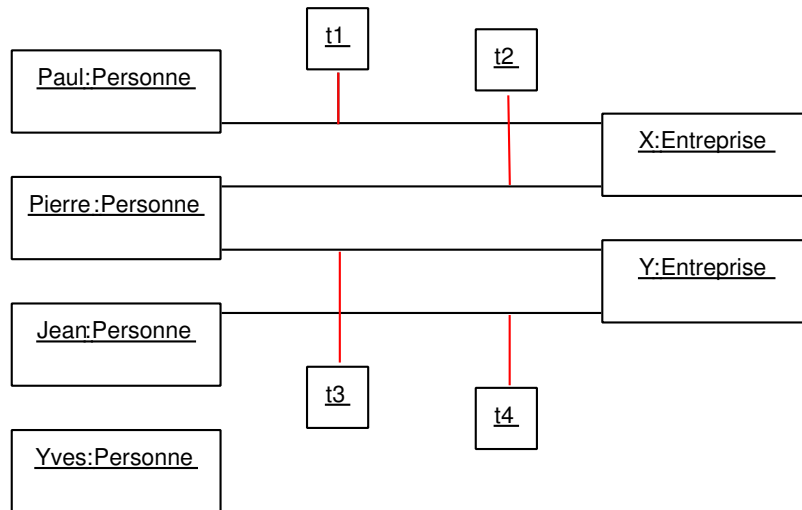
FIG. II. 30 – Diagramme d'objets correspondant au diagramme de classes D_1
