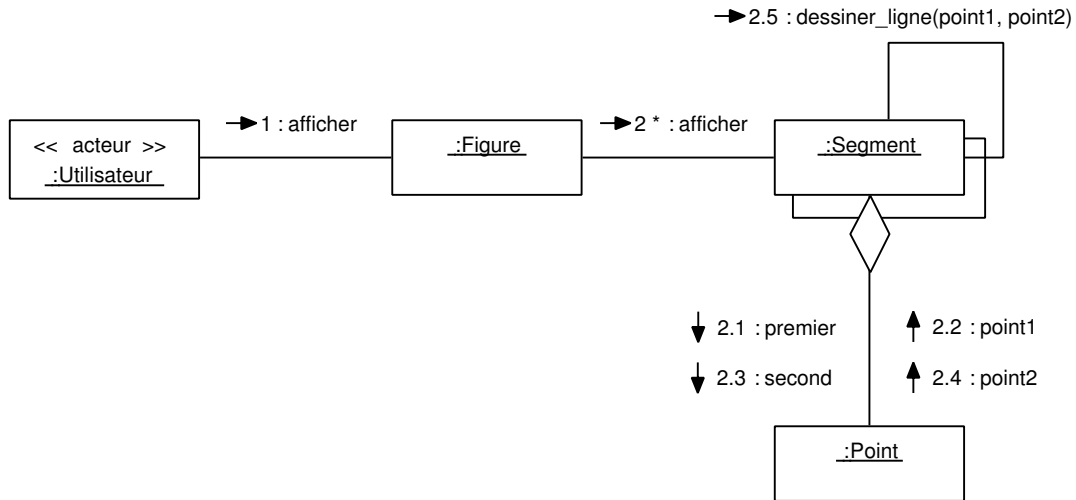
FIG. II. 60 – Diagramme de collaboration représentant l'affichage d'une figure
