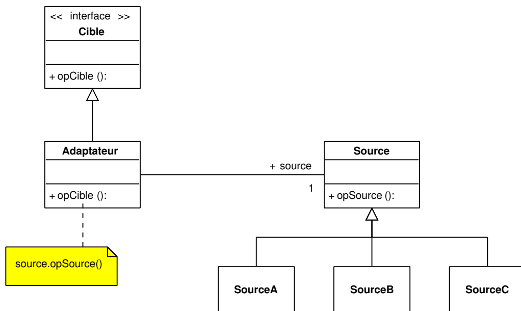
FIG. V. 5 – Patron Adaptateur, par délégation
