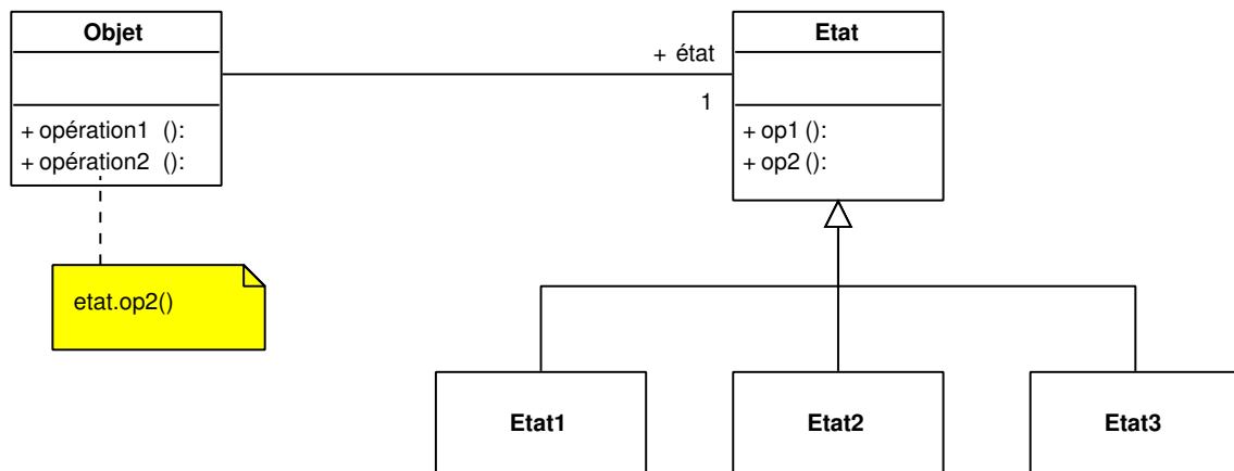
FIG. V. 10 – Patron État
