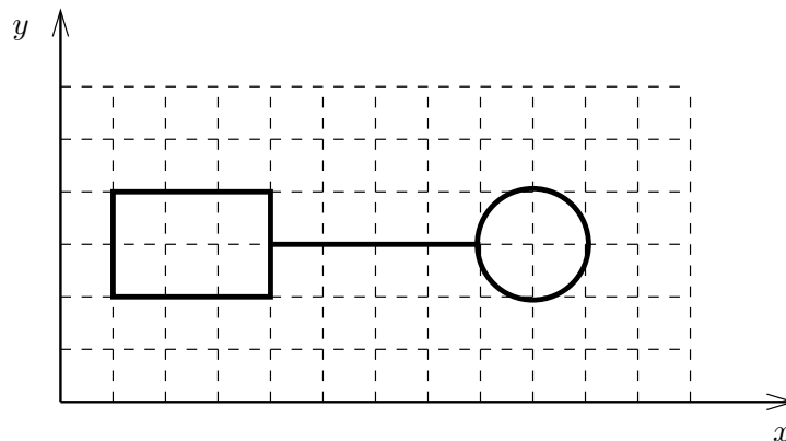
FIG. VI. 26 – Figure géométrique
