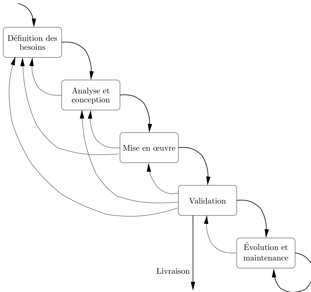
FIG. I. 2 – Modèle incontrôlable
