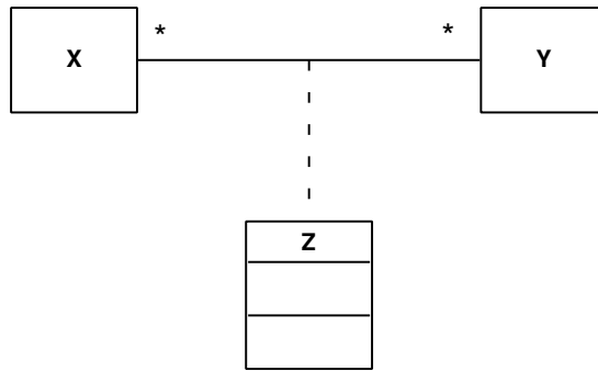
FIG. VI. 30 – Une classe-association
