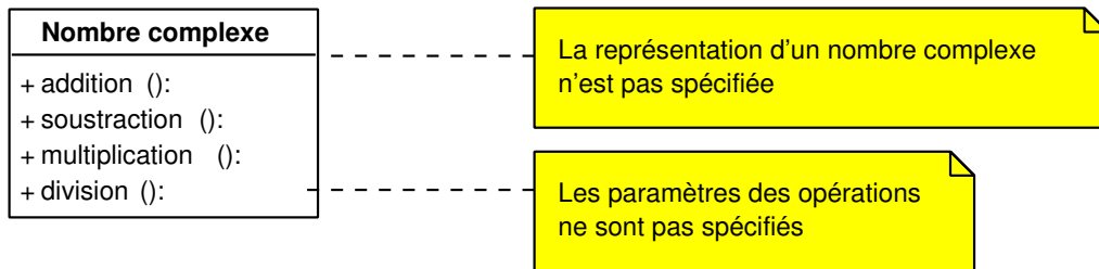
FIG. II. 12 – Classe des nombres complexes ; implantation non précisé
