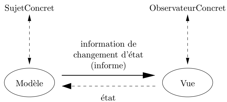
FIG. V. 13 – Implémentation d'une architecture MVC à l'aide du patron Observateur
