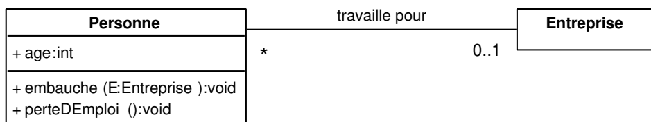
FIG. II. 65 – Diagramme de classes qui représente l'emploi des personnes
