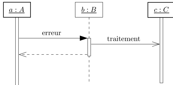
FIG. II. 58 – Les objets a et c sont actifs
