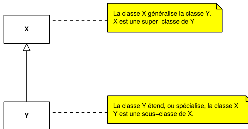
FIG. II. 42 – La classe Y étend la classe X
