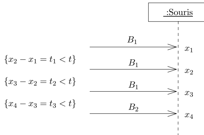
FIG. VI. 27 – Diagramme représentant une séquence de clics
