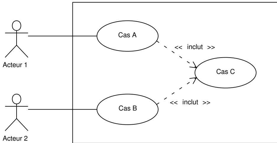
FIG. II. 6 – Limites du système
