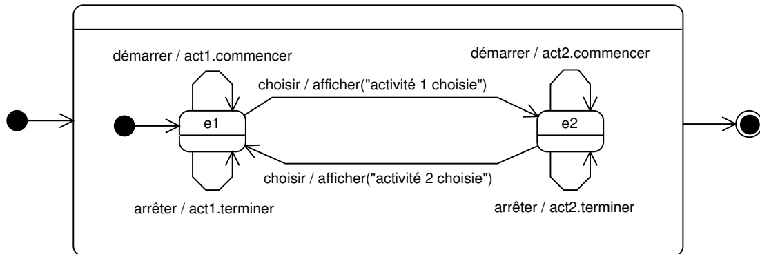
FIG. VI. 22 – Diagramme d'états-transitions de la classe Interface
