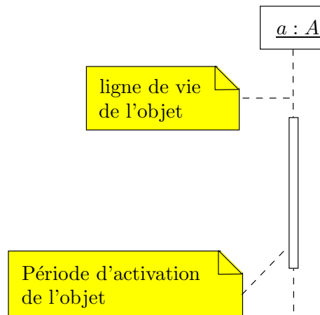
FIG. II. 52 – Période d'activation d'un objet
