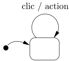
FIG. VI. 28 – Comportement simplifié d'un bouton
