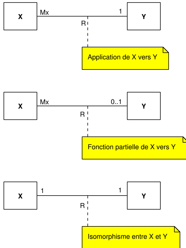
FIG. II. 24 – Cas particuliers d’associations binaires
