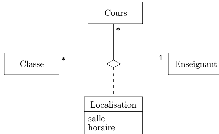
FIG. II. 41 – Relation ternaire entre les classes Cours, Enseignant et Classe
