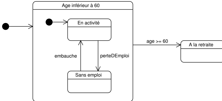
FIG. II. 72 – Exemple d'état composite
