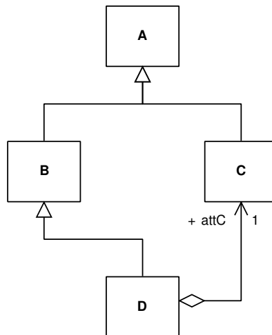
FIG. VI. 15 – Héritage multiple, simulé par délégation
