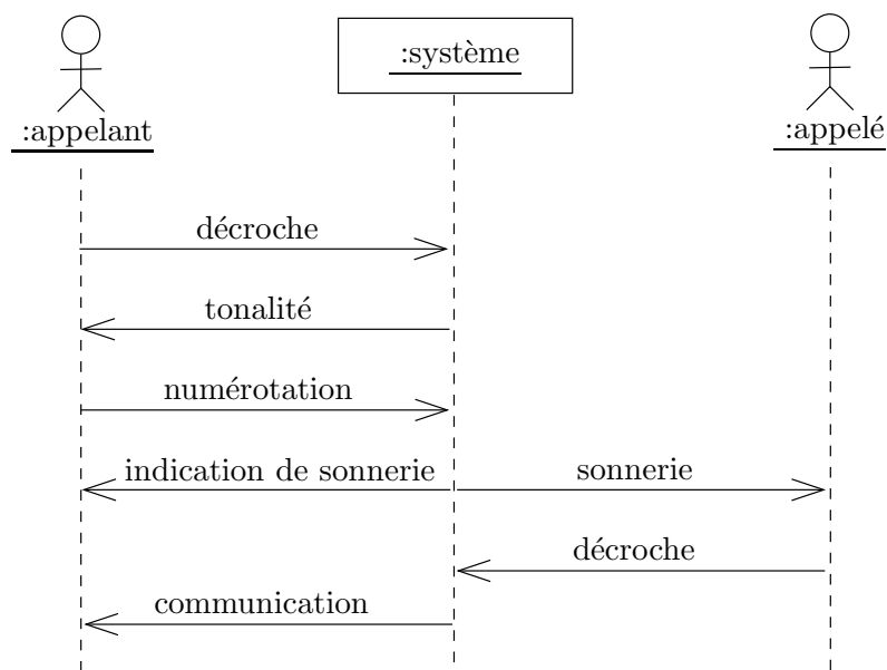
FIG. II. 50 – Diagramme de séquence représentant une communication téléphonique
