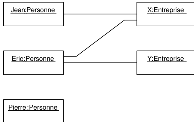
FIG. II. 23 – Diagramme d'objet incorrect par rapport au diagramme de classes figure II. 21
