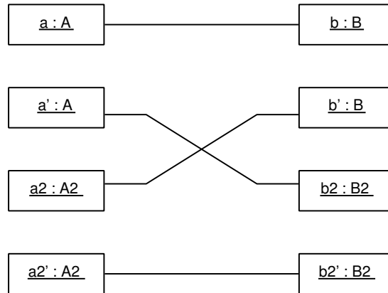
FIG. VI. 12 – Diagramme d’objets correspondant à la figure VI. 11
