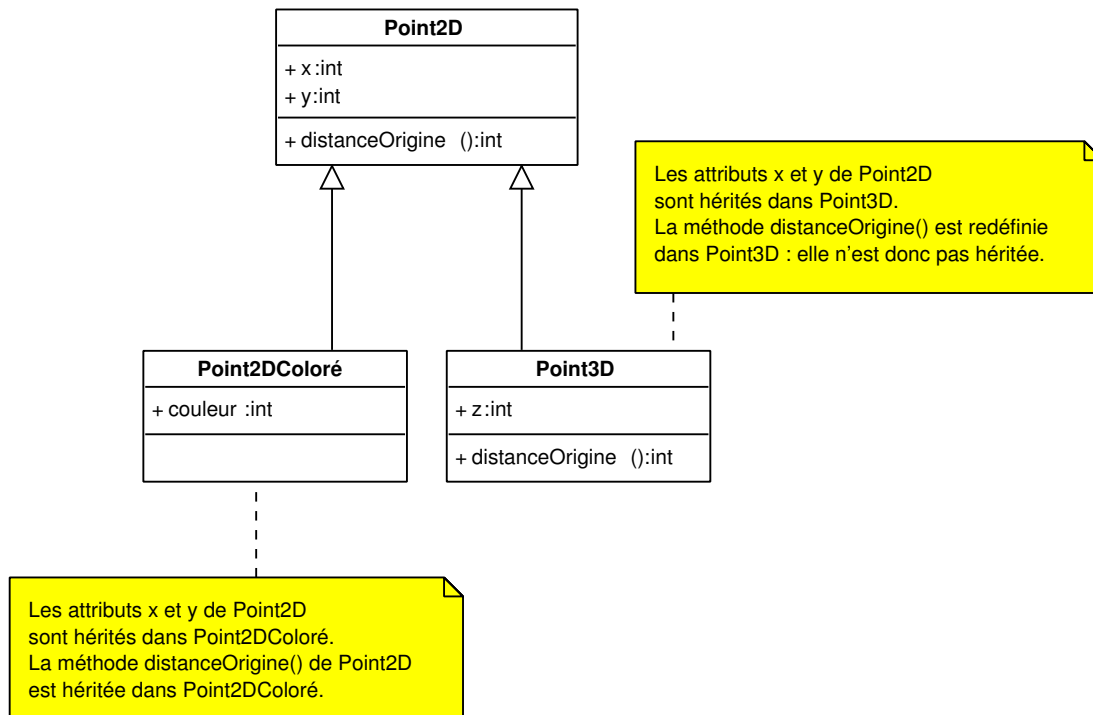
FIG. II. 43 – Diagramme de classes pour des points
