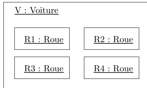
FIG. II. 39 – Représentation équivalente à la figure II. 38
