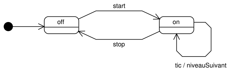
FIG. VI. 18 – Diagramme d'états-transitions de la classe Timer
