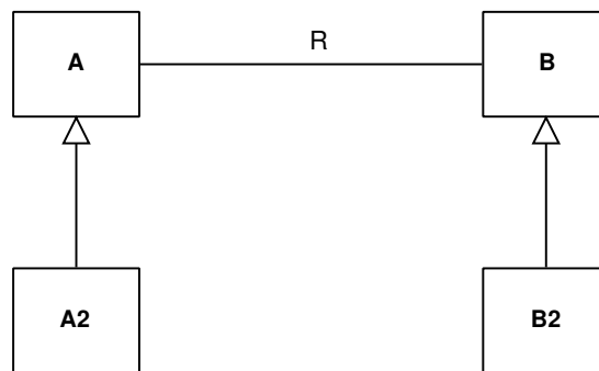
FIG. VI. 11 – Héritage de la relation R
