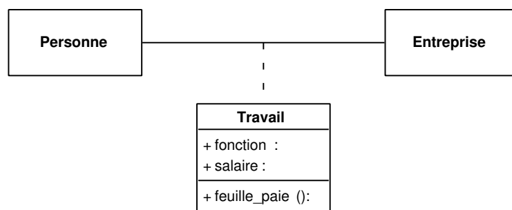
FIG. II. 25 – Exemple de classe-association entre les classes Personne et Travail
