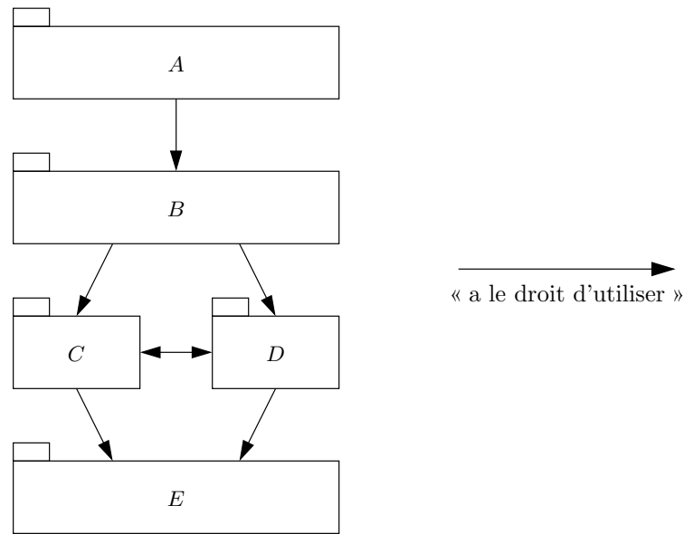
FIG. IV. 3 – Architecture en couches d'une application
