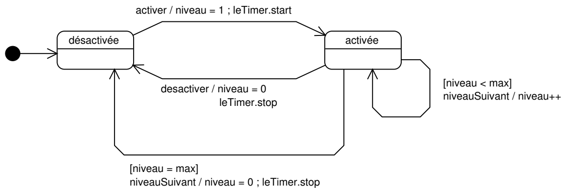
FIG. VI. 19 – Diagramme d'états-transitions de la classe Alarme
