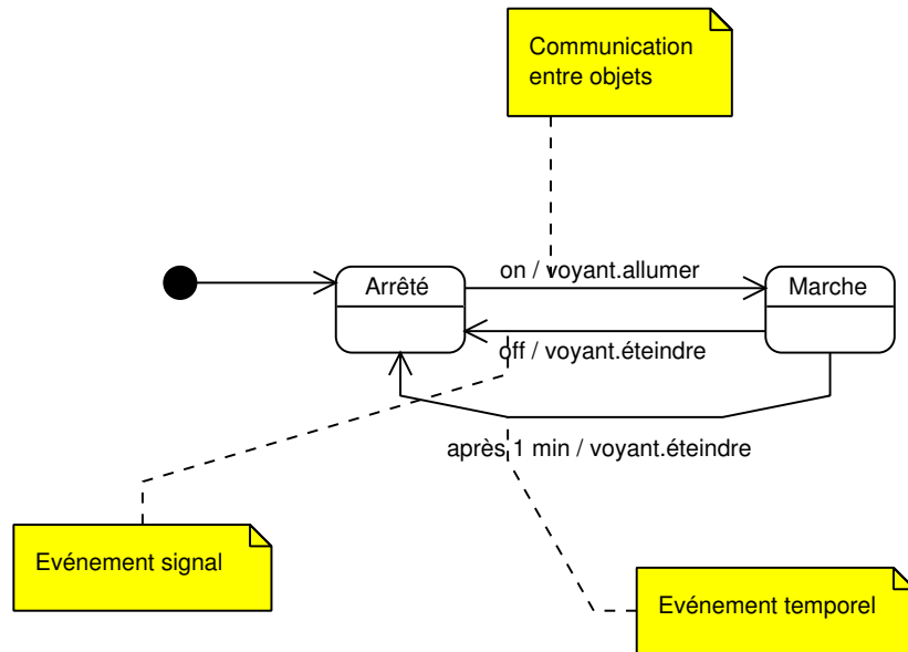
FIG. II. 69 – Diagramme d'états-transitions associé à la classe Machine
