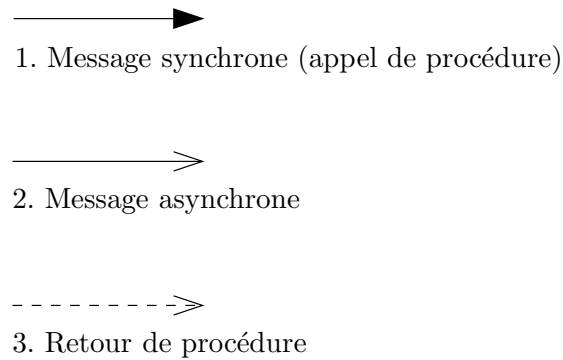
FIG. II. 51 – Les différentes sortes de message
