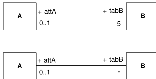
FIG. VI. 9 – Relation avec multiplicité fixée
