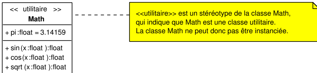
FIG. II. 15 – Classe utilitaire Math
