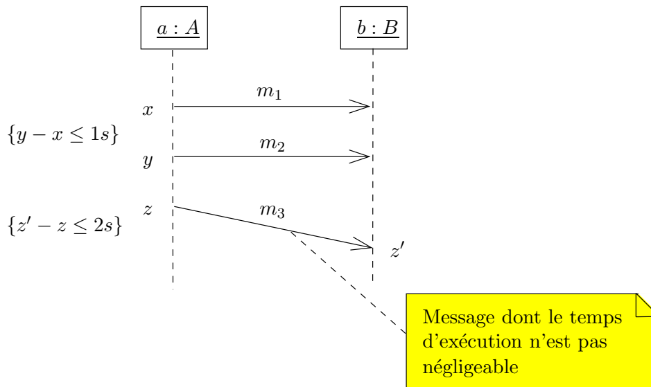
FIG. II. 57 – Contraintes temporelles sur l'envoi et la réception des messages
