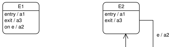
FIG. II. 71 – Action associée à un événement interne et à un événement d'une transition
