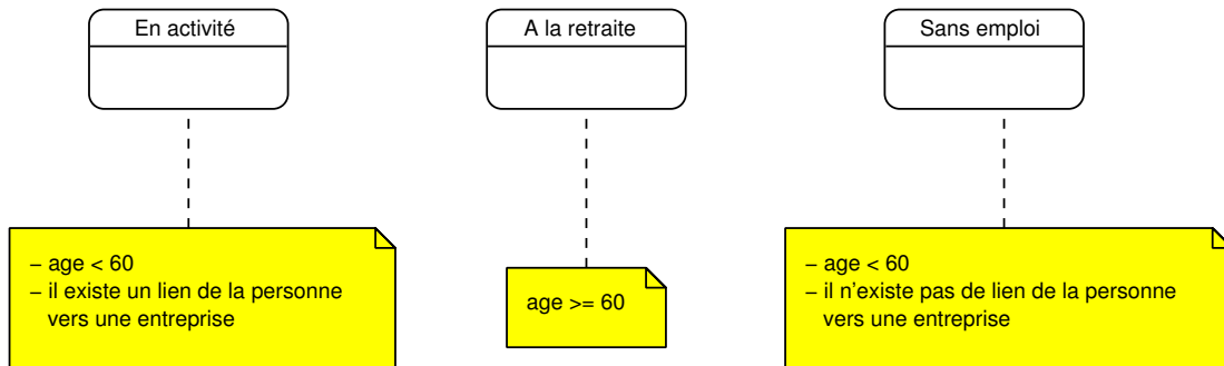
FIG. II. 62 – Trois états possibles pour une personne
