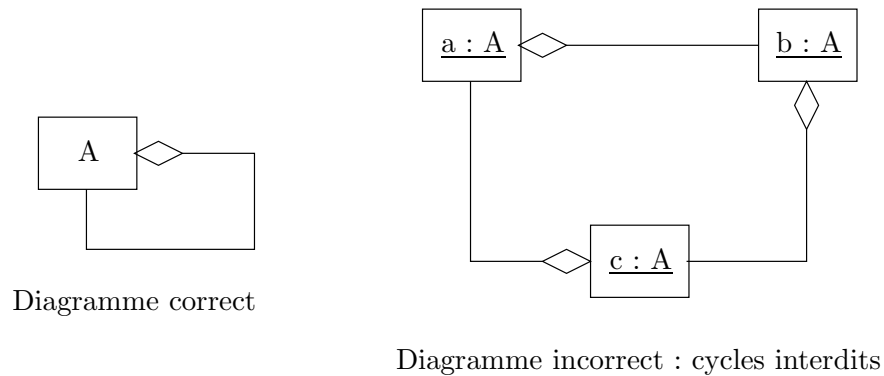
FIG. VI. 13 – Cycles et agrégations
