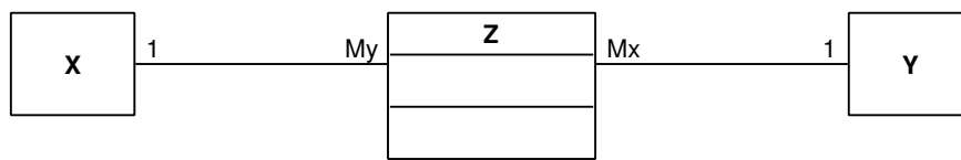
FIG. II. 27 – Simulation d'une classe-association
