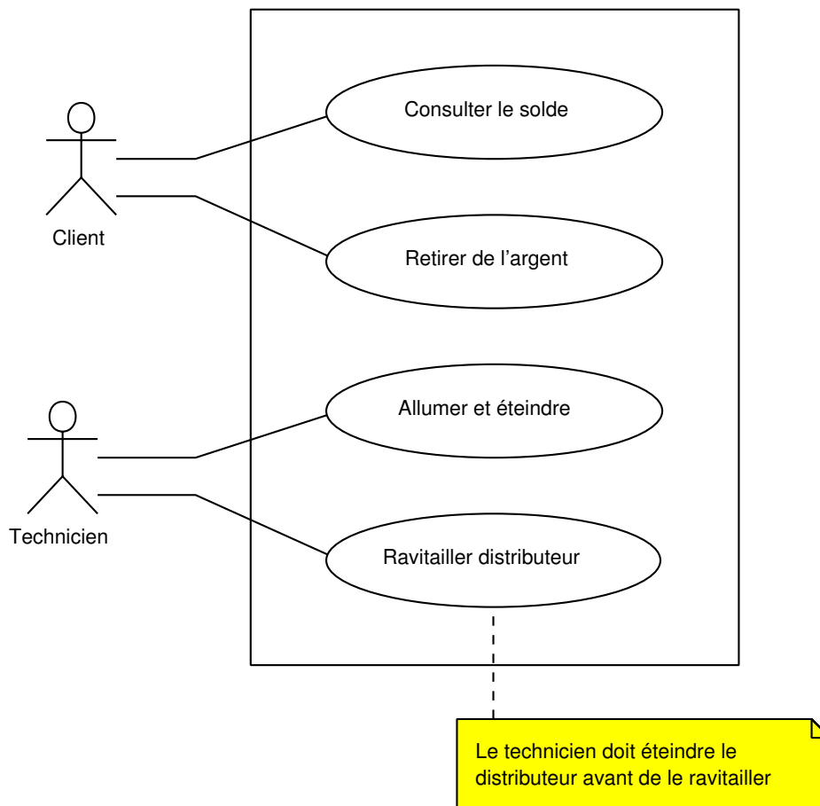
FIG. II. 8 – Diagramme de cas d'utilisation pour un distributeur de billets
