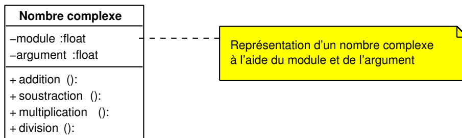
FIG. II. 13 – Classe des nombres complexes ; implantation avec module et argument
