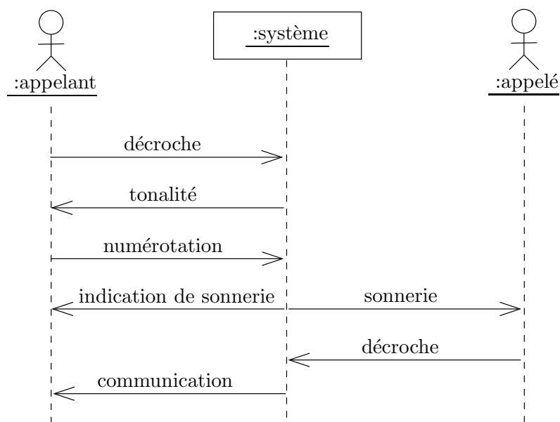
FIG. III. 1 – Diagramme de séquence représentant une communication téléphonique
