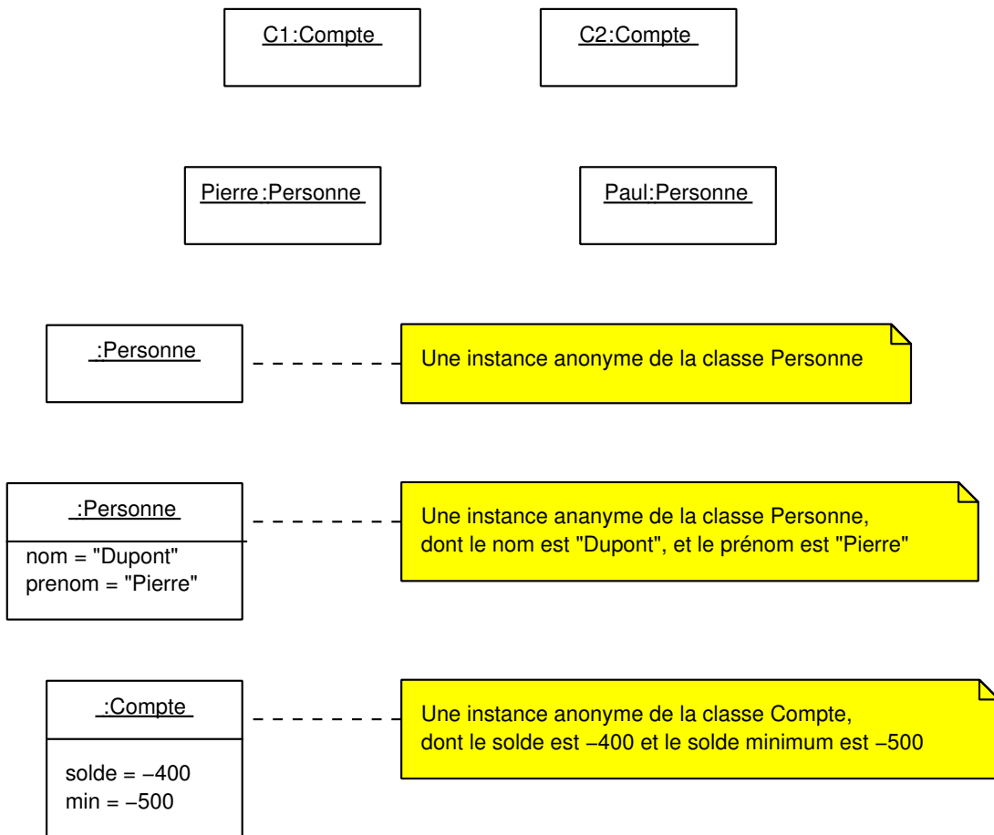
FIG. II. 11 – Exemples d’instances des classes Compte et Personne
