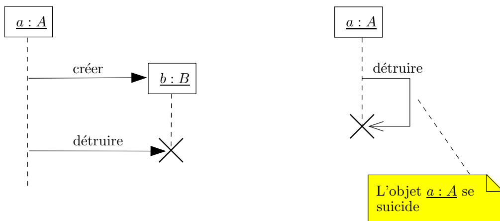
FIG. II. 54 – Création et destruction d’objets
