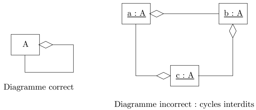
FIG. II. 35 – Cycles et agrégations
