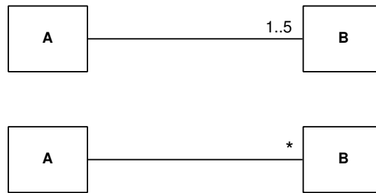
FIG. VI. 5 – Multiplicités de cardinalité variable
