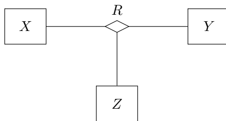
FIG. VI. 31 – Une relation ternaire
