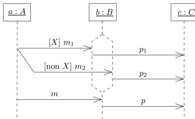
FIG. II. 56 – Dédoublément d'une ligne de vie
