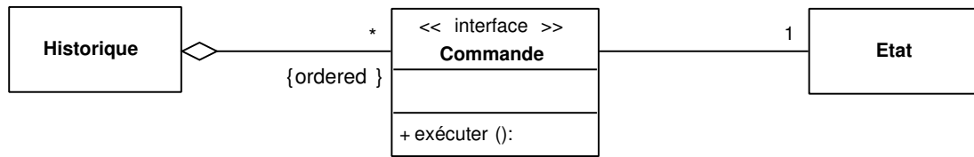
FIG. V. 9 – Historique de commandes
