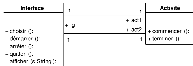
FIG. VI. 21 – Diagramme de classes de l'application permettant d'exécuter deux activités
