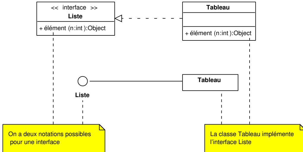
FIG. II. 48 – La classe Tableau implémente l'interface Liste
