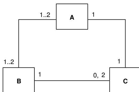
FIG. VI. 24 – Diagramme de classes de l'exercice 4
