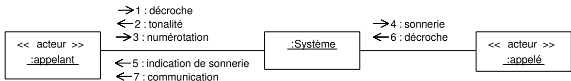
FIG. II. 59 – Diagramme de collaboration représentant une communication téléphonique
