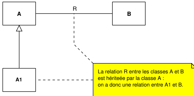
FIG. II. 45 – La relation R est hérité par A_1
