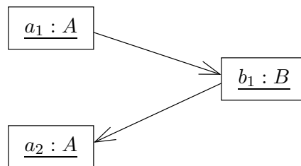
FIG. VI. 7 – Liens incohérents
