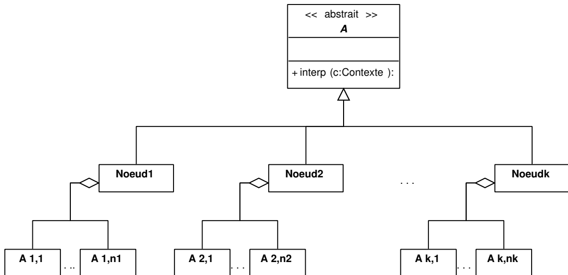
FIG. V. 14 – Patron Interprète
