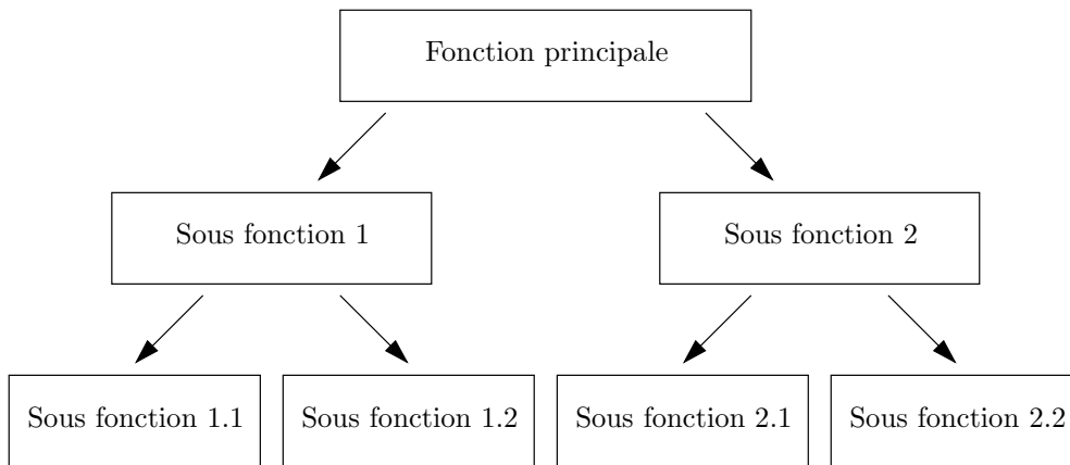
FIG. I. 7 – Décomposition fonctionnelle
