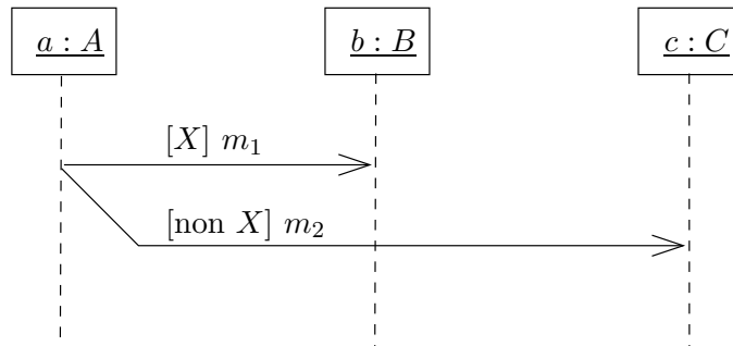
FIG. II. 55 – Messages conditionnels
