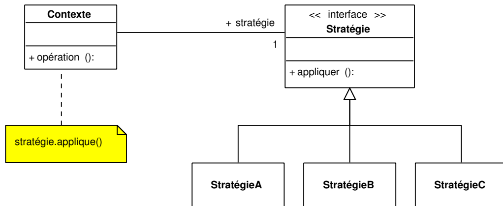
FIG. V. 6 – Patron Stratégie
