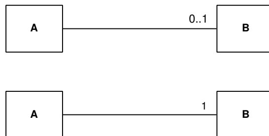
FIG. VI. 3 – Multiplicités simples
