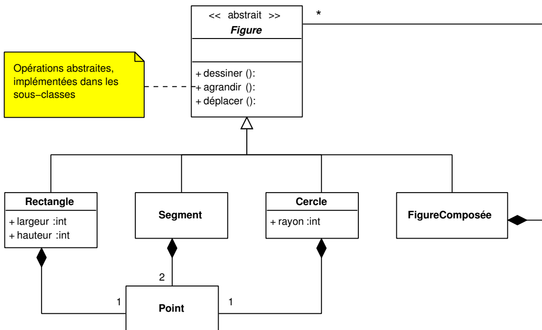
FIG. V. 3 – Figures géométriques
