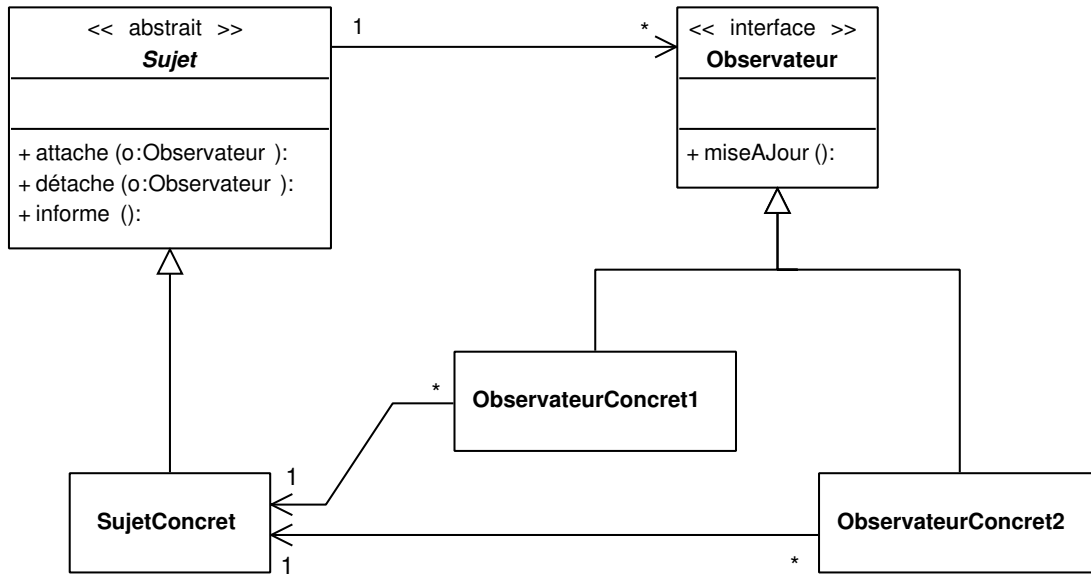
FIG. V. 12 – Patron Observateur
