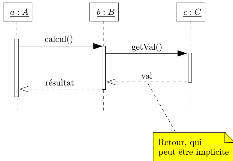
FIG. II. 53 – Périodes d’activation lors d’appels de procédure
