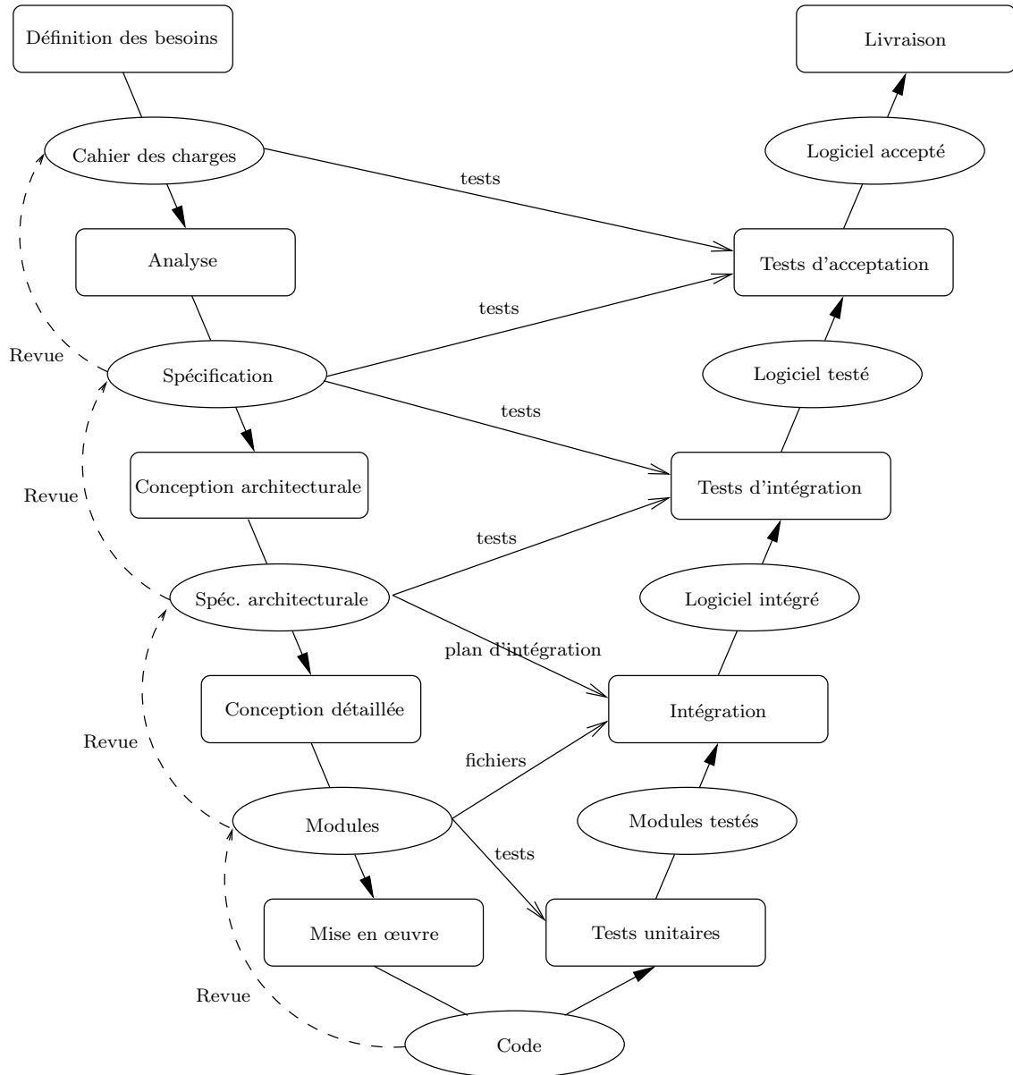
FIG. I. 3 – Modèle du cycle de vie en V
