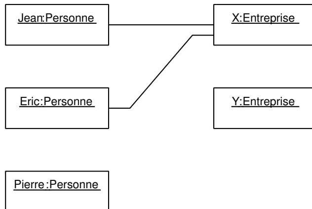
FIG. II. 22 – Diagramme d'objet correct par rapport au diagramme de classes figure II. 21
