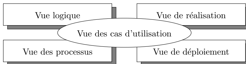
FIG. IV. 1 – Le modèle des 4 + 1 vue de Philippe Kruchten
